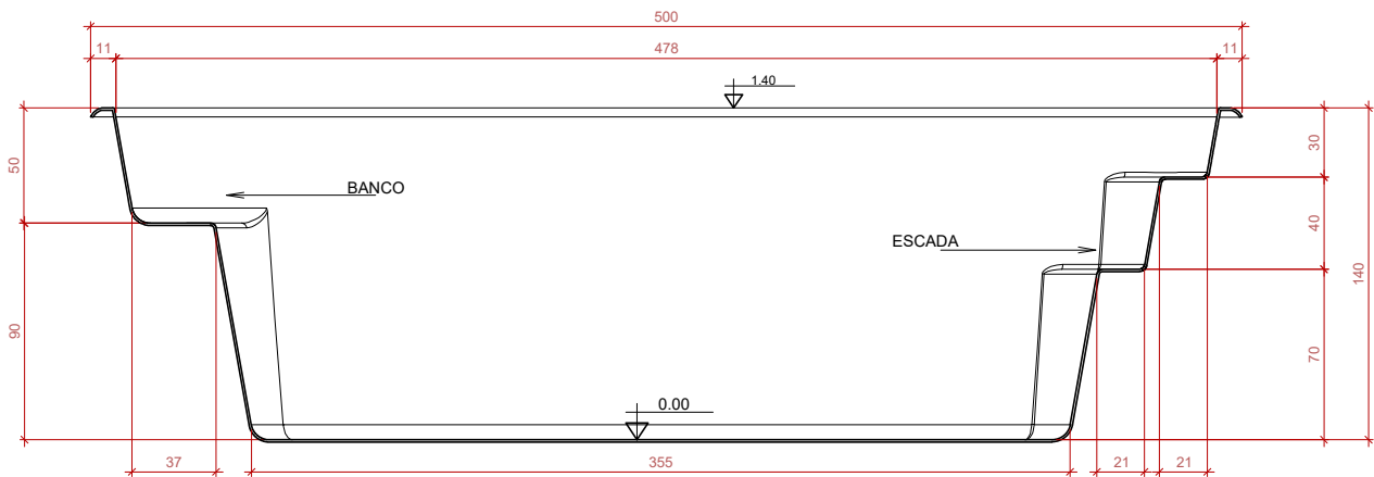
CORTE LONGITUDINAL SEM ESCALA
